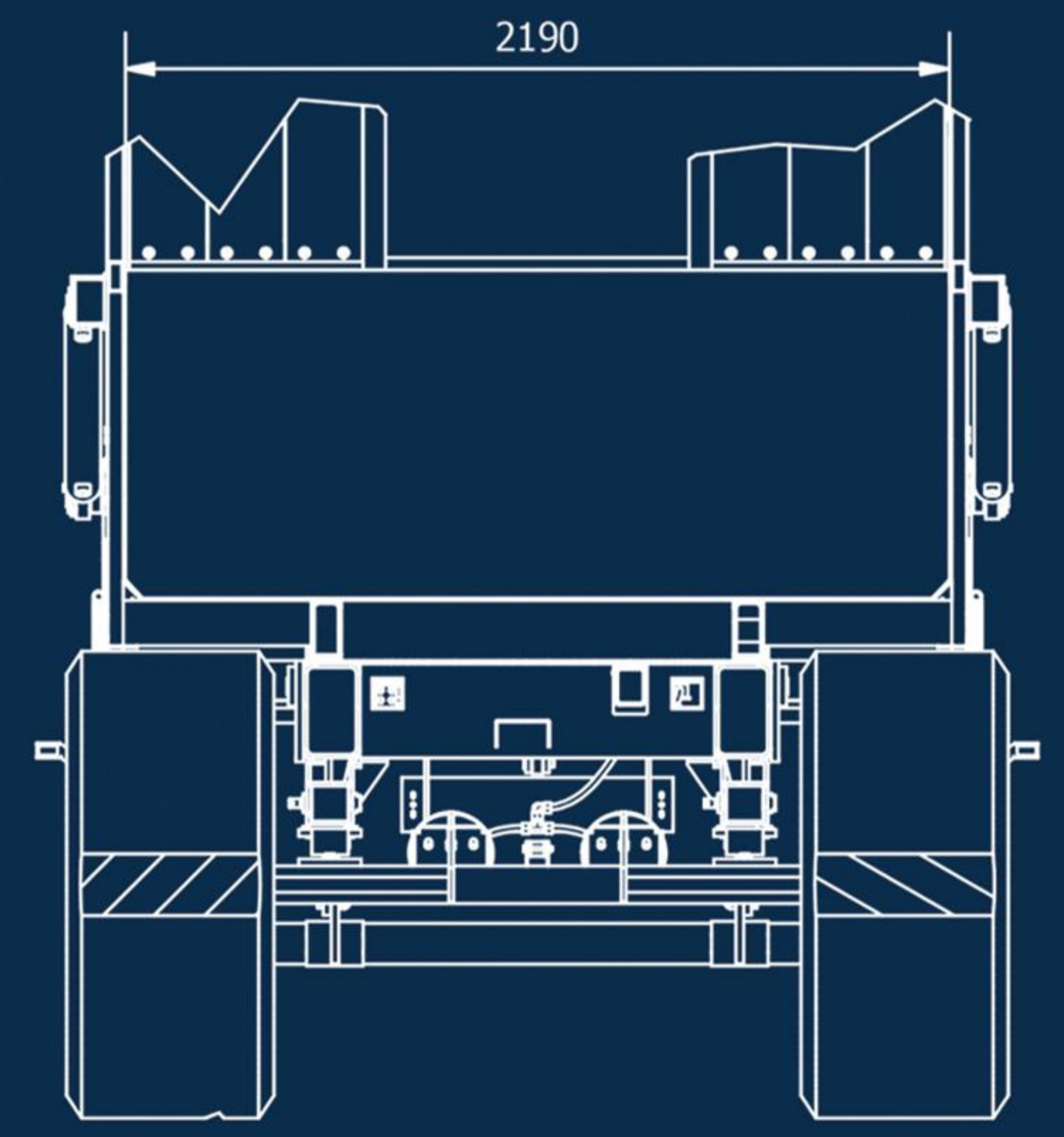
E-E ( 1 : 30 )
