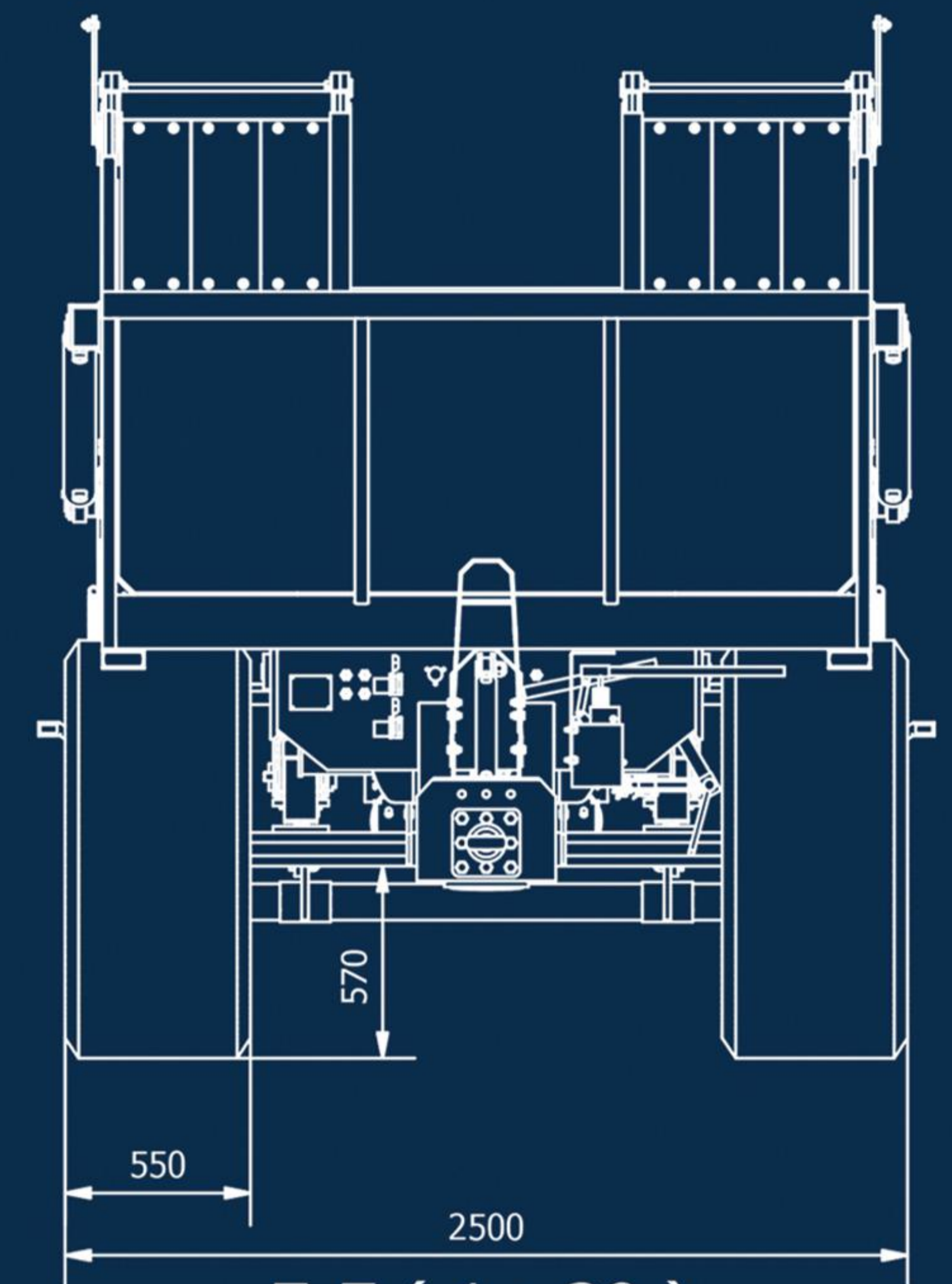
E-E ( 1 : 30 )
